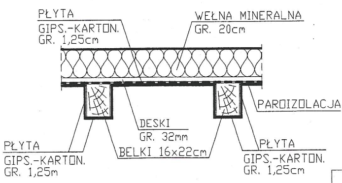
OBICIE BELEK STROPOWYCH PŁYTAMI KIPSOWO-KARTONOWYMI DETAL "A" SKALA 1:25
